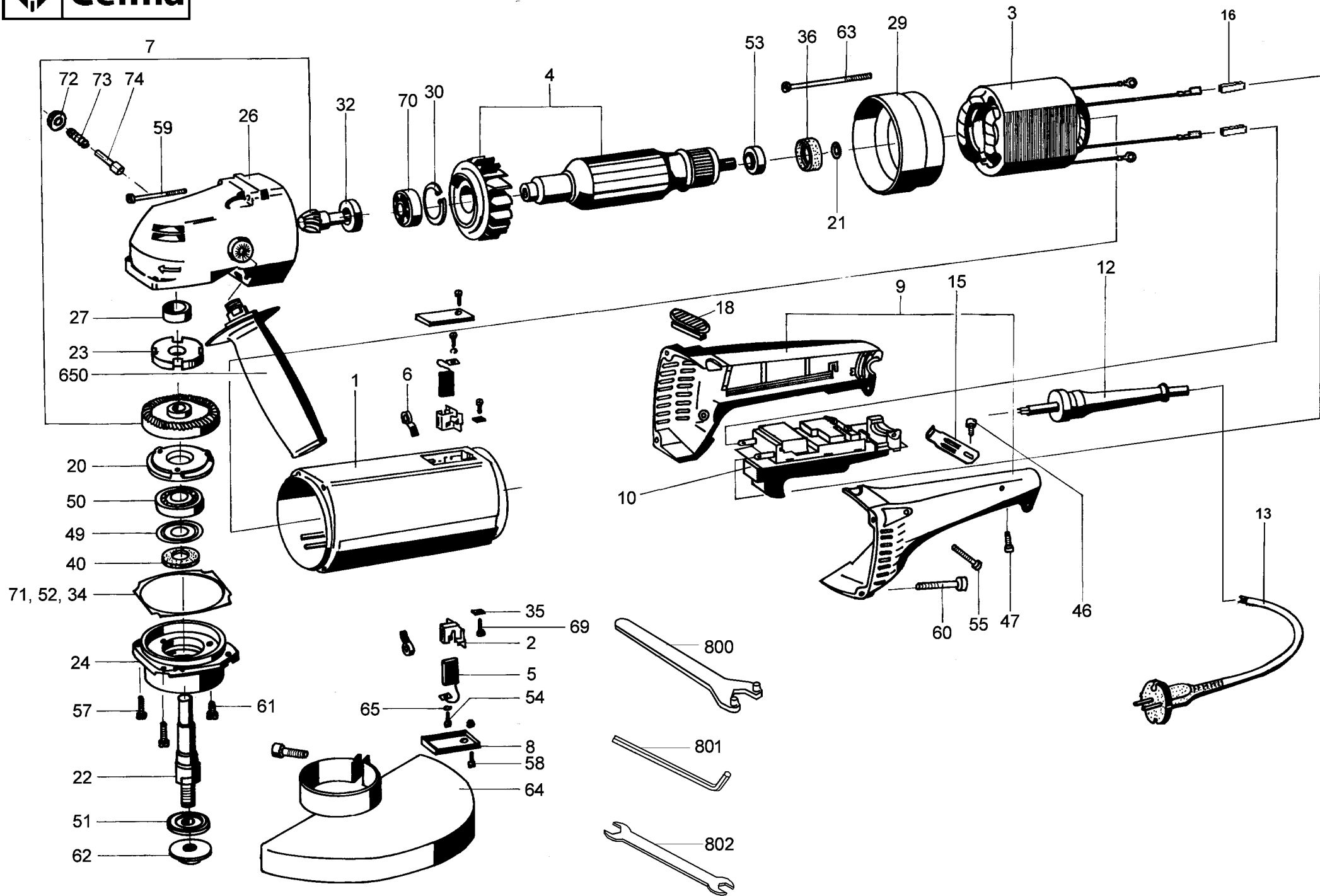
Szlifierka kątowna obwodowa PRAg 230BR
