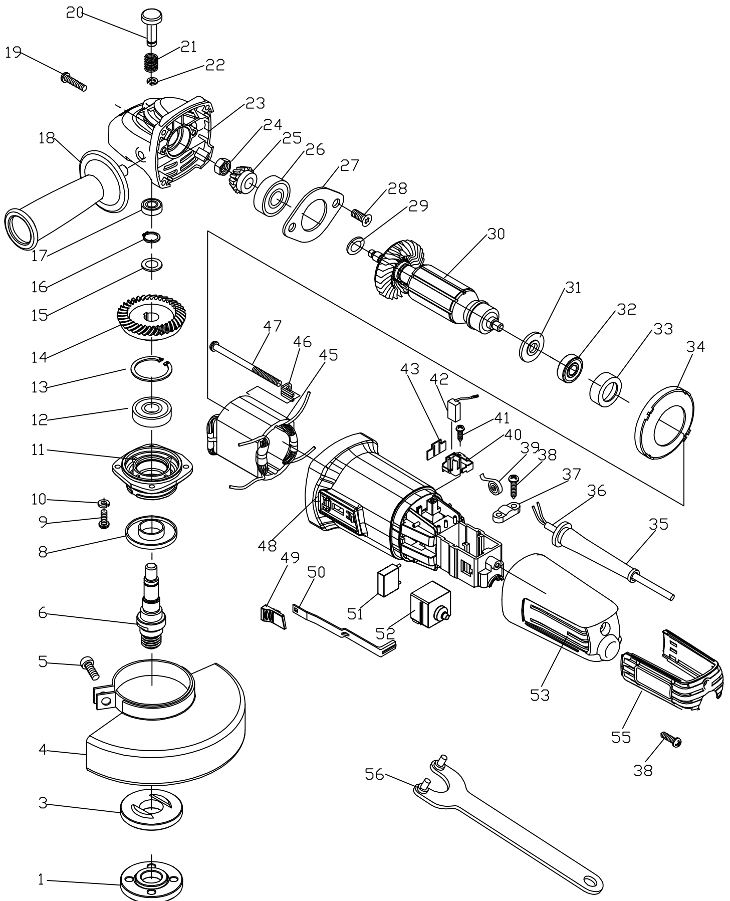
Szlifierka kąтова obwodowa PRAG 125A
