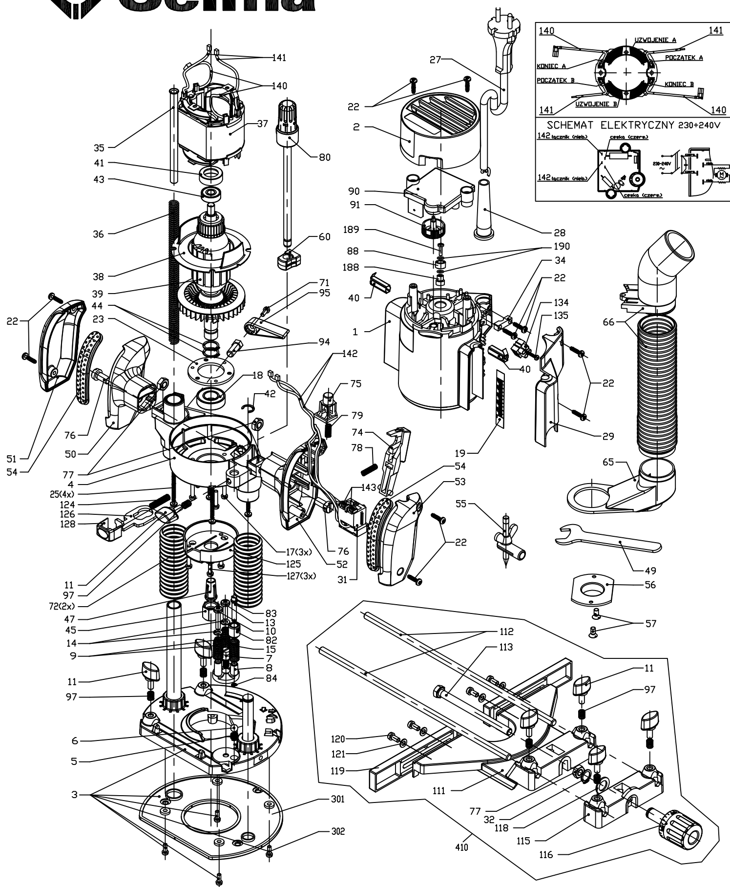
Frezarka DFRa 8ES
