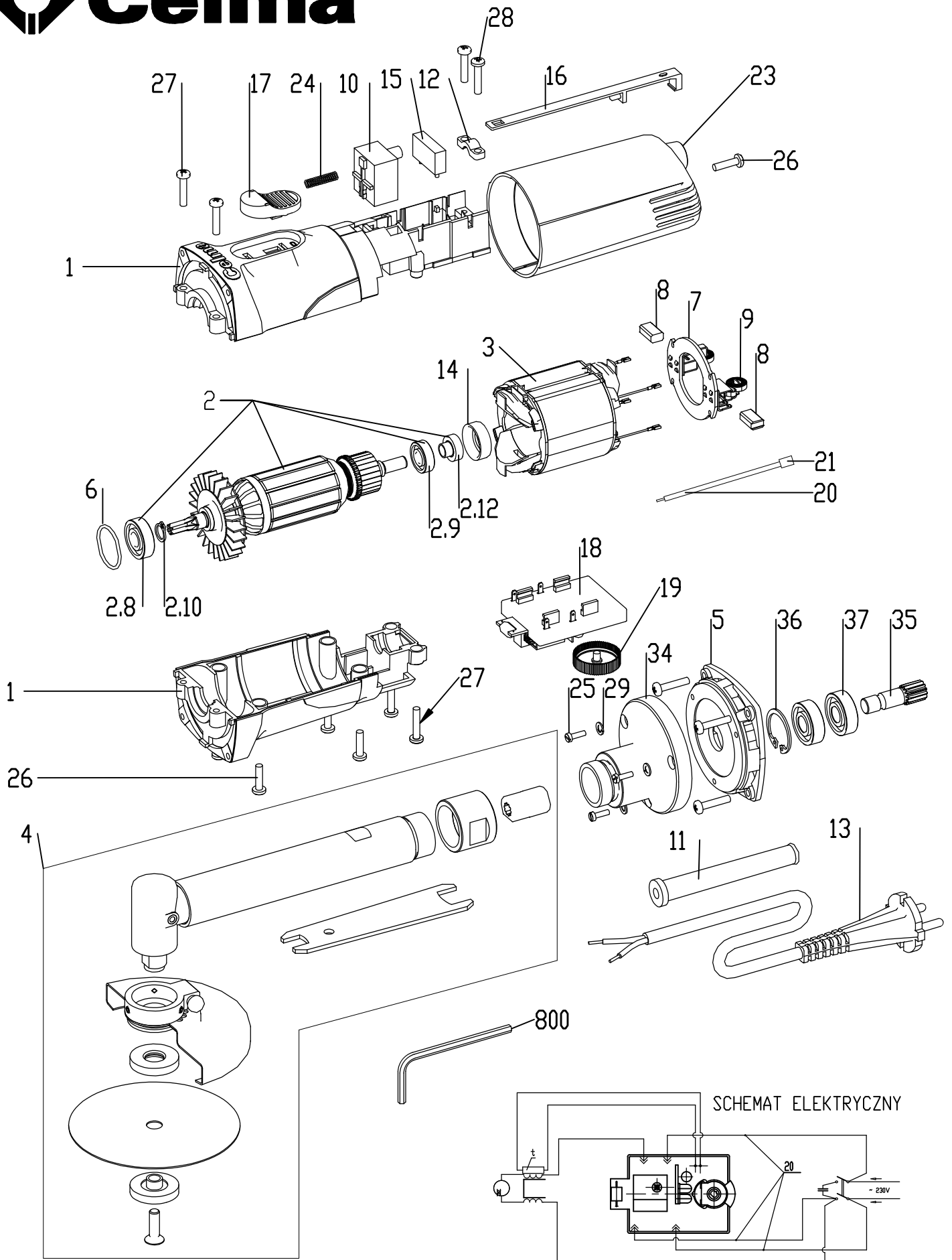
Szlifierka kątowna przedłużona PRAg 4ES
