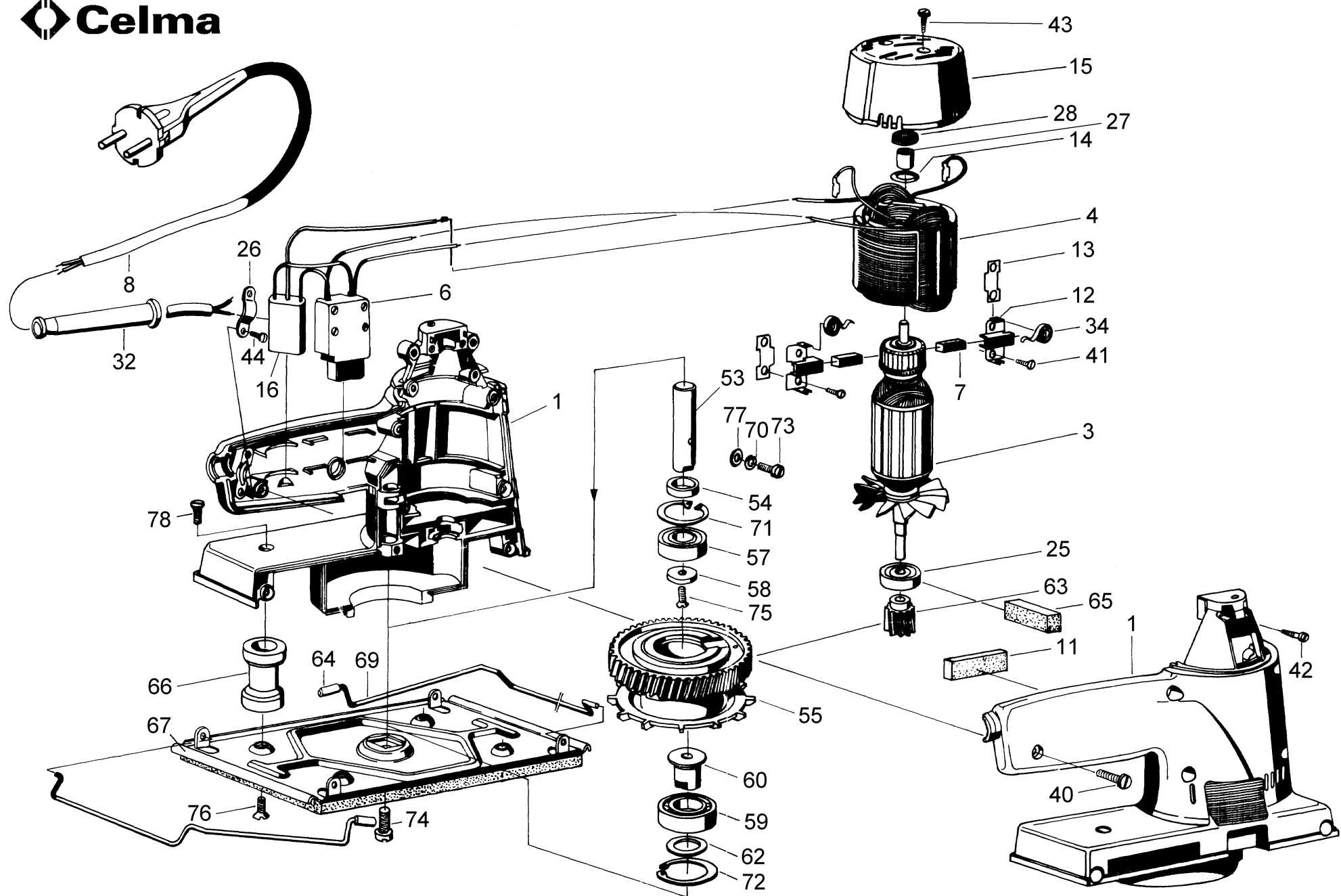
Szlifierka oscylacyjna DBSSw 114IIB
